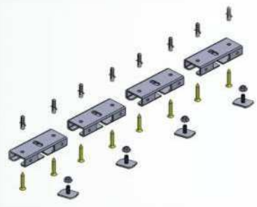
95313.01 KIT PARED conjunto de 4 escuadras suspensión en aplique MAGNET.
